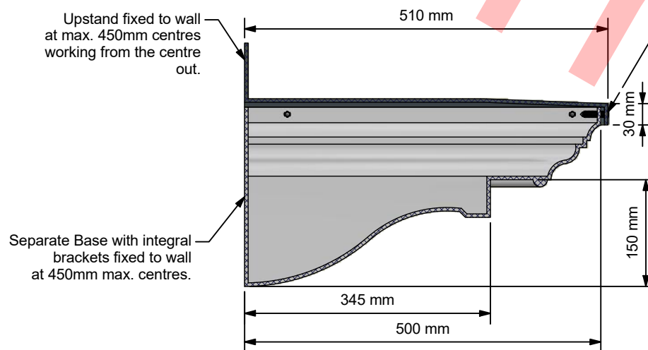
A-A ( 1:7.5 )
