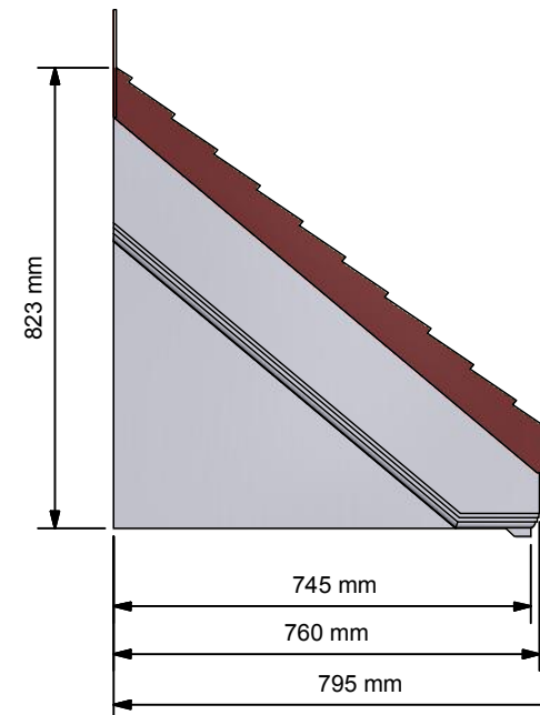
Side Elevation ( 1:15 )
