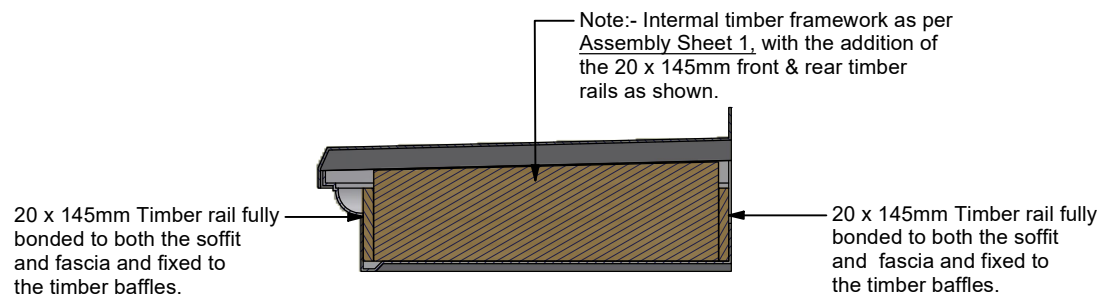
A-A ( 1:15 )
