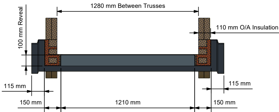
B-B ( 1 : 20 )
