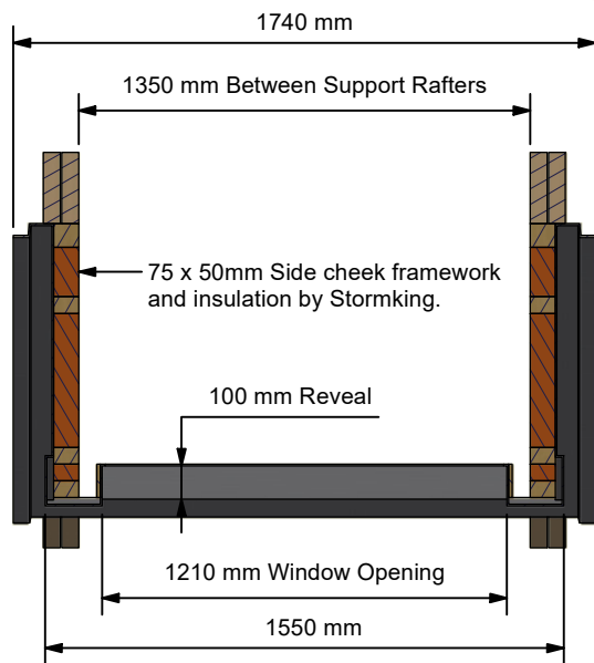
B-B ( 1:25 )
