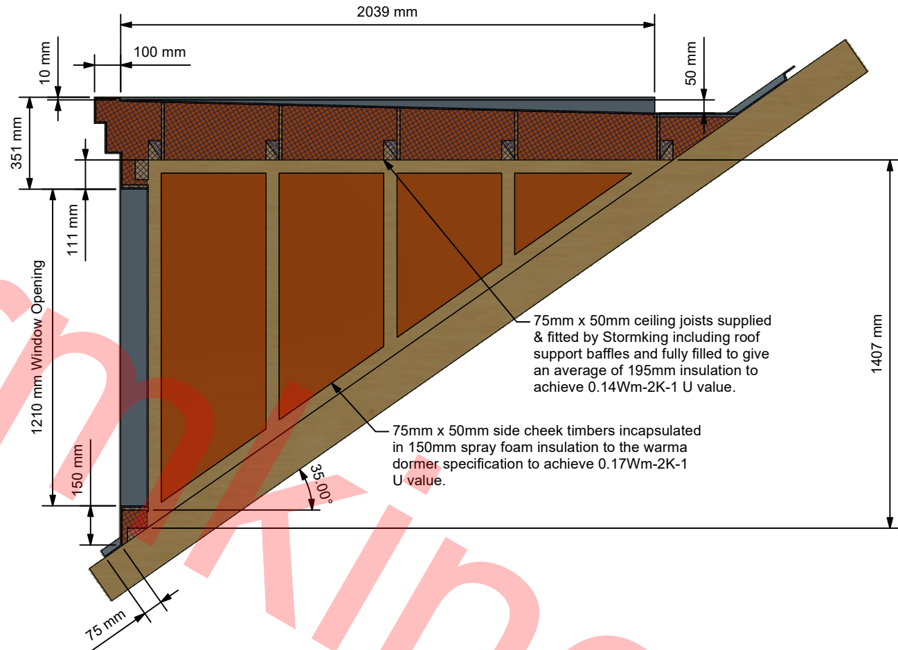
A-A ( 1 : 20 )
