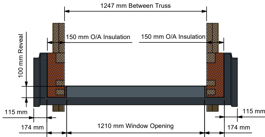
B-B ( 1 : 20 )
