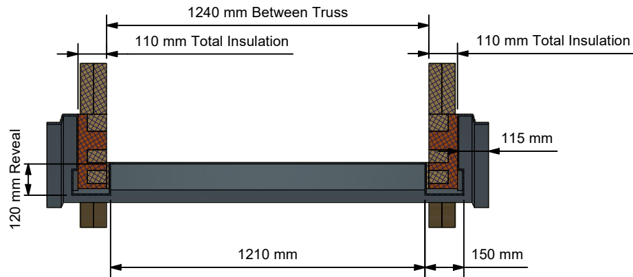
B-B ( 1 : 20 )
