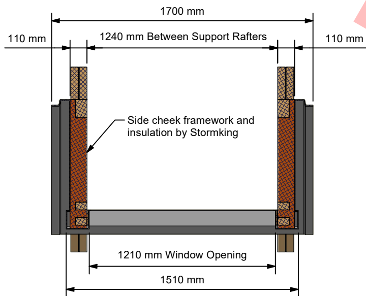
A-A ( 1:25 )
