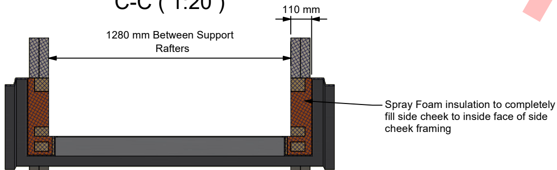
C-C ( 1:20 )
