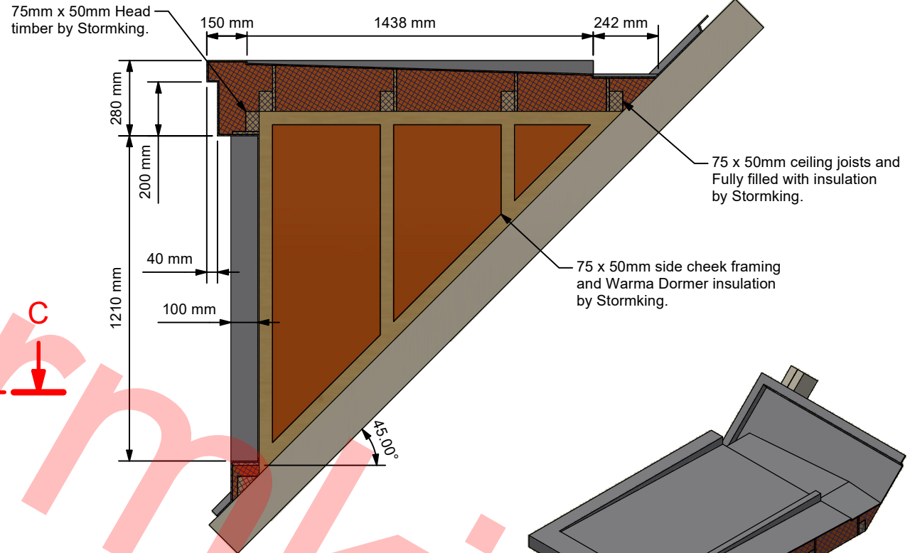
D-D ( 1:20 )
