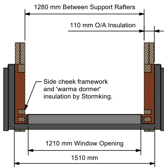
A-A ( 1:25 )
