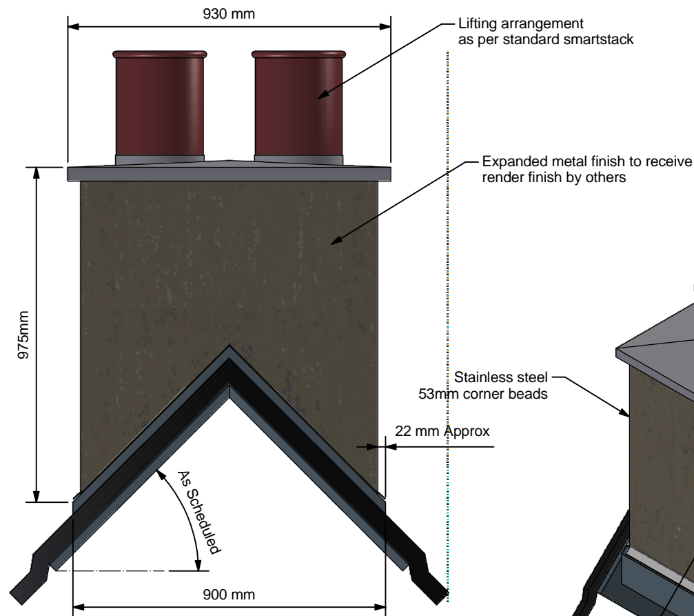
Side Elevation ( 1:15 )
