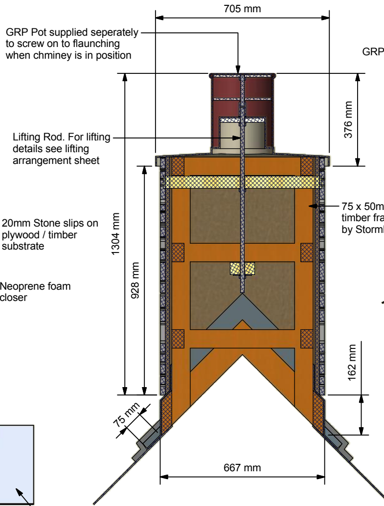
A-A ( 1:15 )
