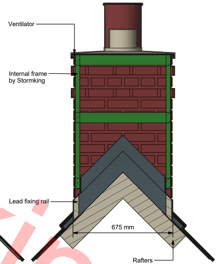
Section A-A ( 1 : 15 )
