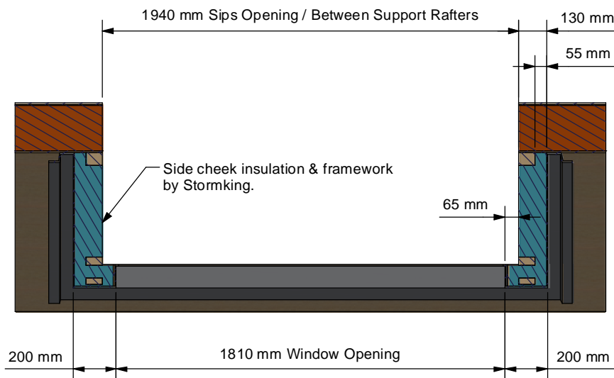
B-B ( 1:25 )
