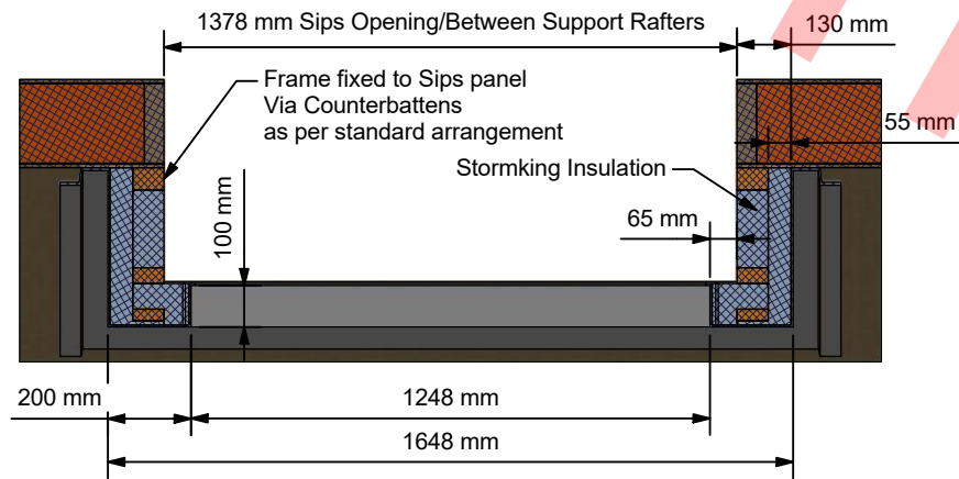
B-B ( 1:20 )
