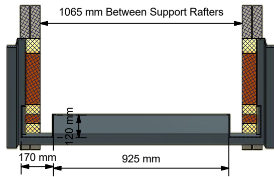
C-C ( 1:20 )
