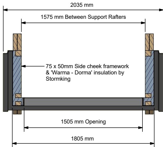
B-B ( 1 : 25 )
