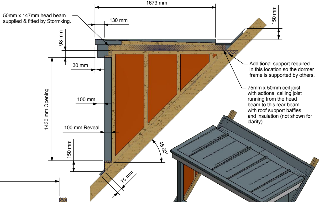
A-A ( 1 : 25 )
