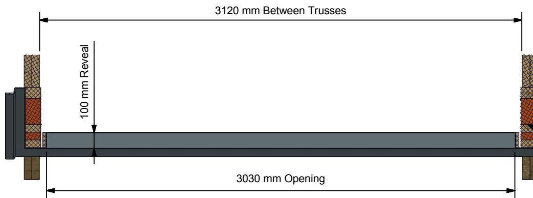
B-B ( 1 : 25 )
