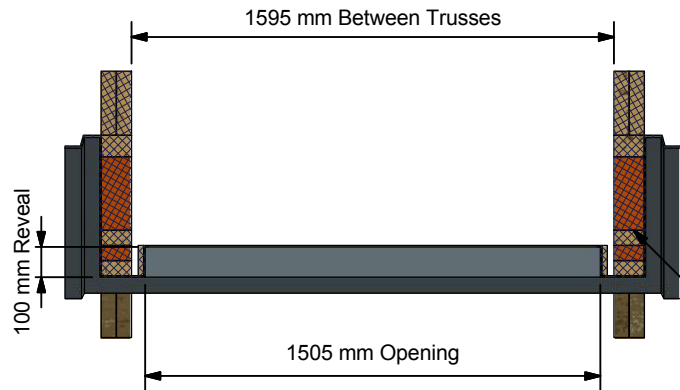
B-B ( 1 : 25 )
