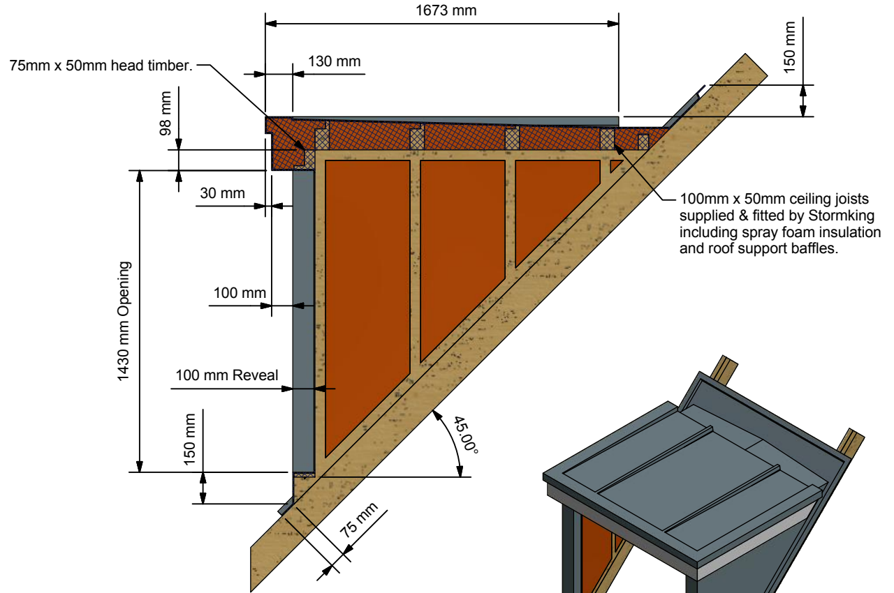
A-A ( 1 : 25 )
