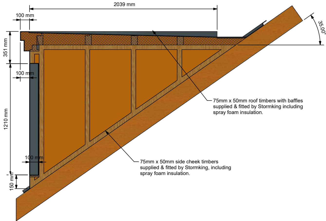
Section A-A ( 1 : 20 )
