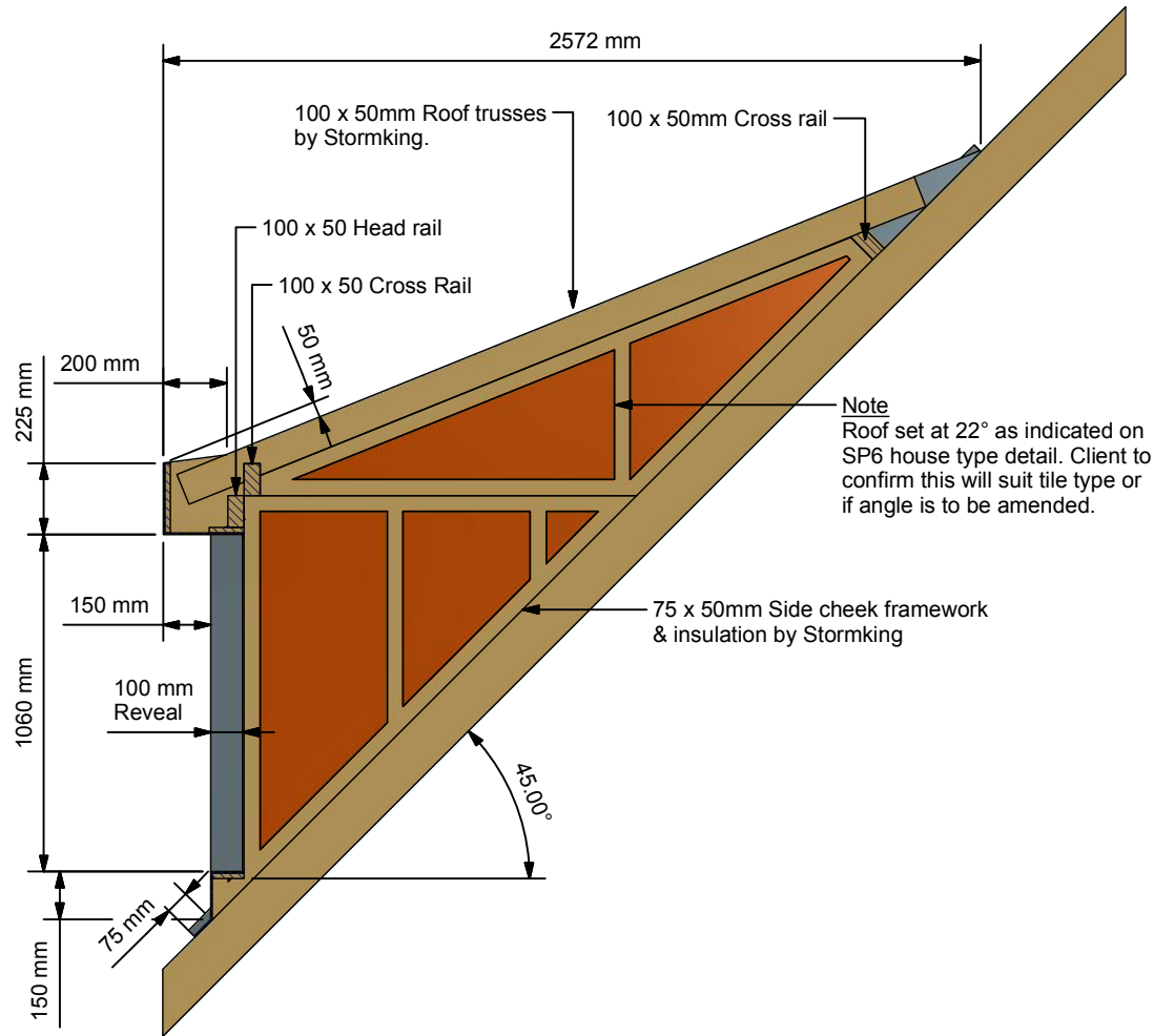
A-A ( 1:25 )
