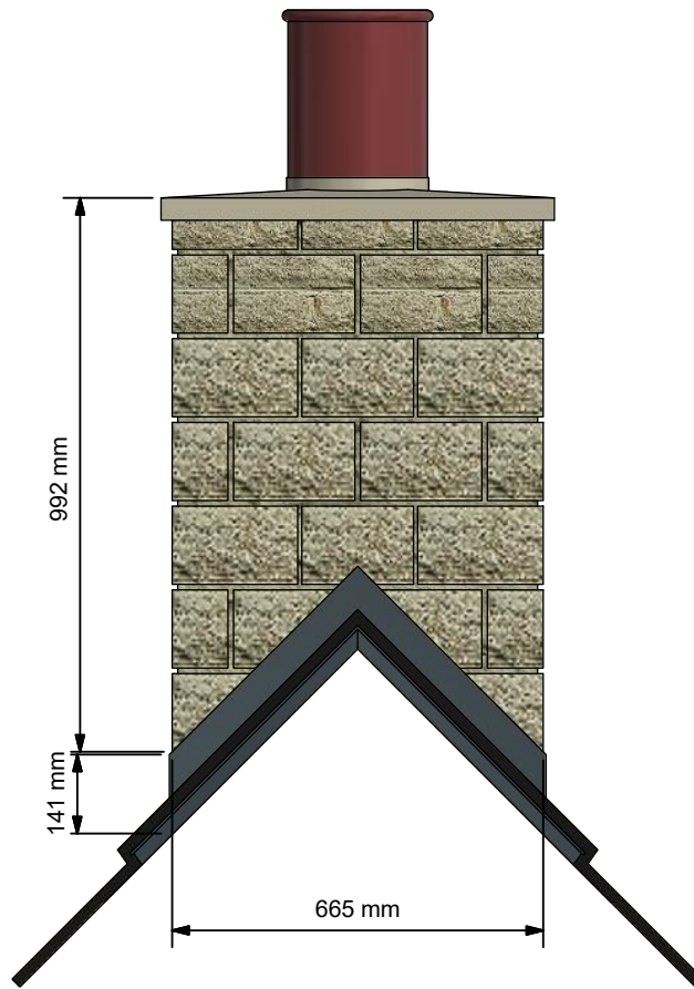
Side Elevation ( 1:15 )
