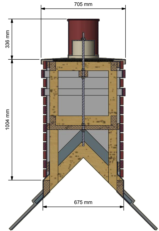
Section A-A ( 1:15 )
