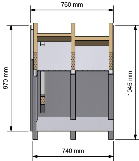
A-A ( 1:20 )
