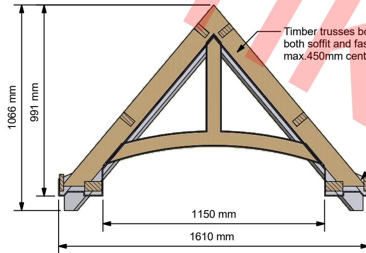
B-B ( 1:20 )
