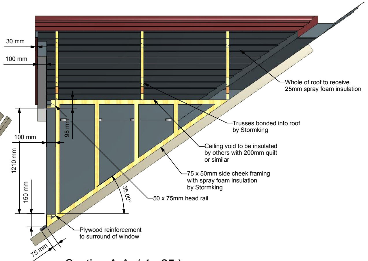
Section A-A ( 1 : 25 )
