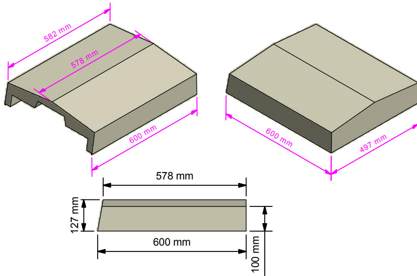
Side View Stop End/Base Mitre ( 1 : 15 )
