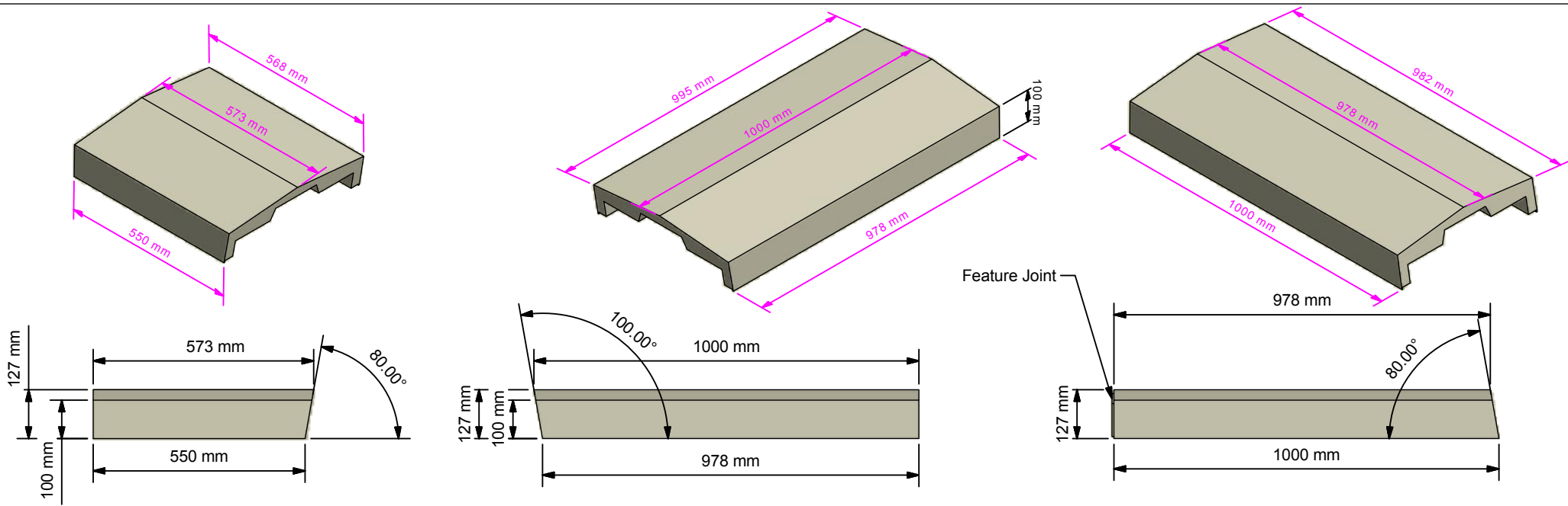
Side View - Top Mitre ( 1 : 15 ) Side View Top Mitre Straight ( 1 : 15 ) Side View Bottom Mitre Straight ( 1 : 15 )
