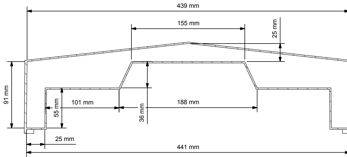
B-B ( 1 : 3 )
