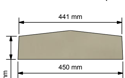
Stop End ( 1 : 10 )
