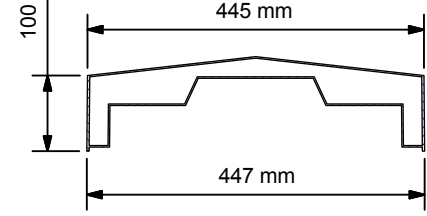
Section A-A ( 1 : 10 )
