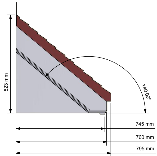
Side Elevation ( 1:15 )
