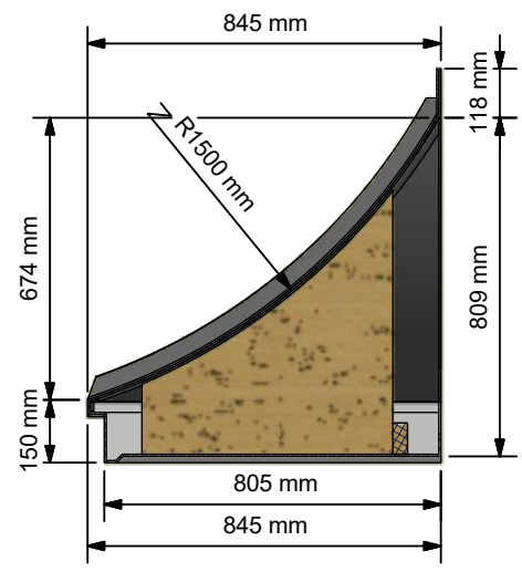
A-A ( 1:20 )
