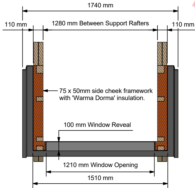
B-B ( 1:25 )
