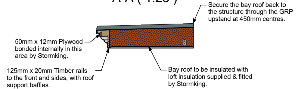
A-A ( 1:25 )
