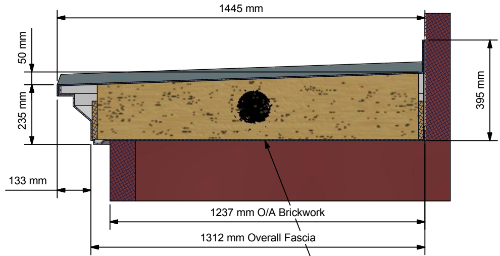
A-A ( 1 : 15 )
