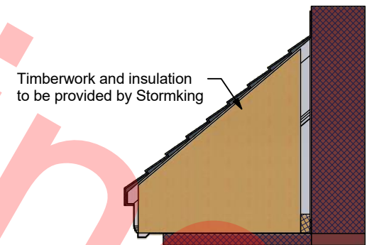
A-A ( 1 : 20 )
